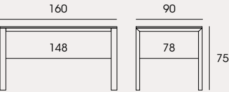
GOLTAY 160x90 + 1 ext.60 / 2 ext.50
