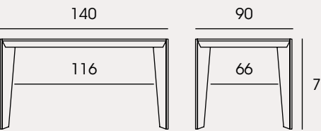
STELA 140x90 + 1 ext.60
