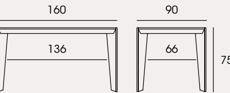
STELA 160x90 + 1 ext.60 / 2 ext.50
