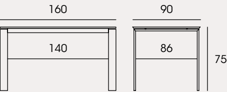
ALIENA 160x90 + 1 ext.60
