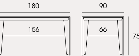
STELA 180x90 + 1 ext.60 / 2 ext.50
