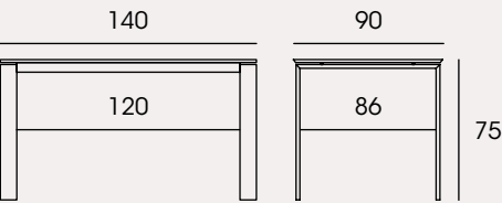
ALIENA 140x90 + 1 ext.60
