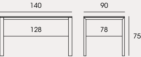
GOLTAY 140x90 + 1 ext.60 / 2 ext.45
