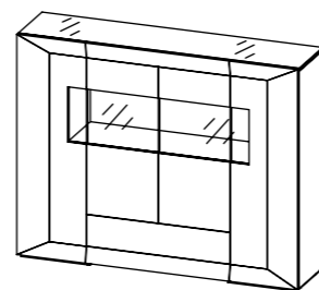
VG7 Móvel Vitrina 4 Portas, 1 Gaveta T. Vidro Cód 2110A12.. C 1800 H 1420 P 428
