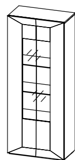
VG5 Móvel Vitrina 2 Portas Vidro Cód P2141A12.. C 800 H 1950 P 428
