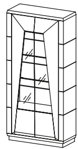
DM2 Móvel Vitrina 2 Portas H.2000 CÓD P2199A15.. C 950 H 2000 P 440
