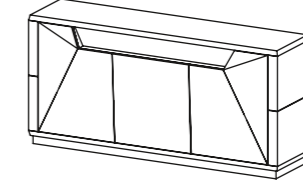
DM5 Aparador 3 Portas, 1 Gaveta C.2100 CÓD P1426A15.. C 2100 H 1000 P 540
