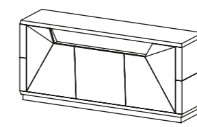
DM5 Aparador 3 Portas, 1 Gaveta C.2000 CÓD P1425A15.. C 2000 H 900 P 540
