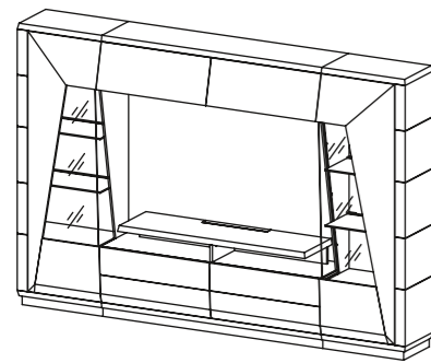
DM1 Estante TV C.3000 CÓD P3806A15.. C 3000 H 2000 P 480
