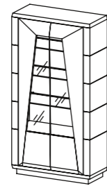
DM4 Móvel Vitrina 2 Portas H.1800 CÓD P2161A15.. C 950 H 1800 P 440
